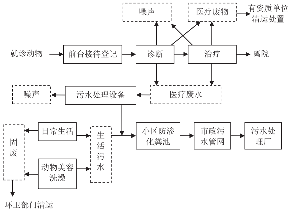
图 3 运营期工艺流程及产污环节
