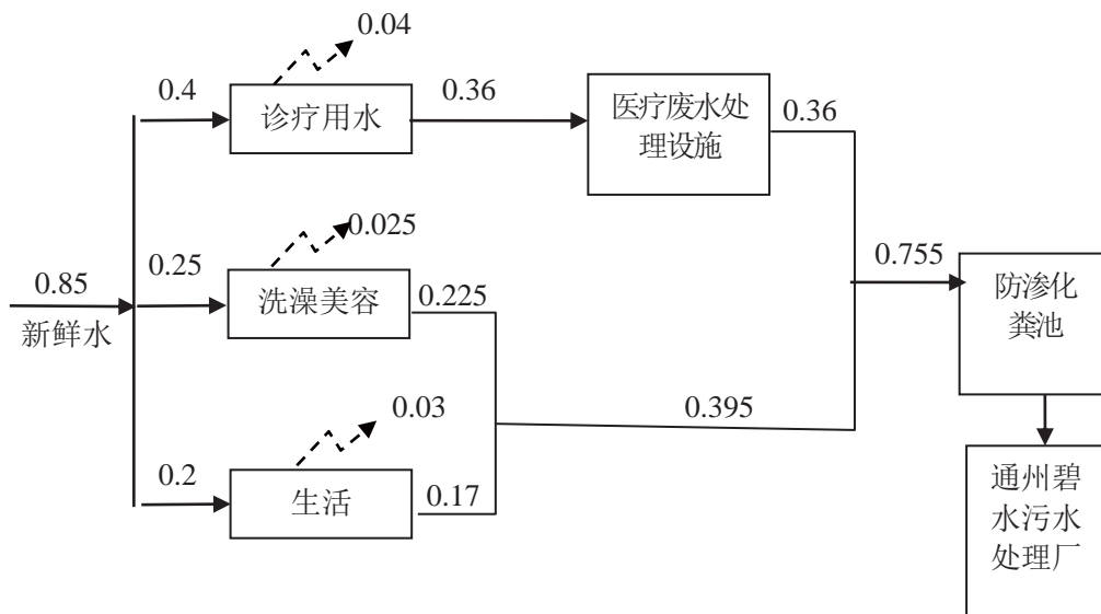
图 3 水平衡图 单位：m 3 /d
